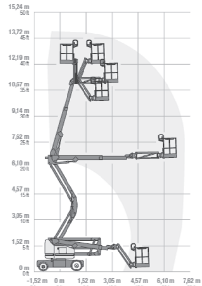
Arbeitsdiagramm des Korbarms Z-40/23N RJ
