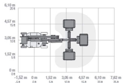
Arbeitsdiagramm des Korbarms Z-40/23N RJ
